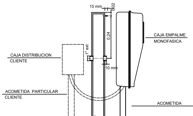
DETALLE A FIJACION
